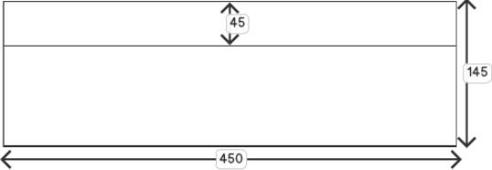
Окно Уведомления
