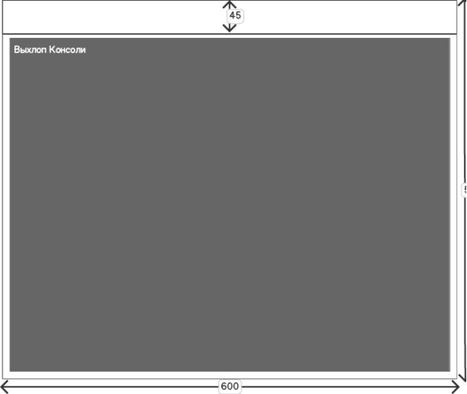
Окно Консоли
