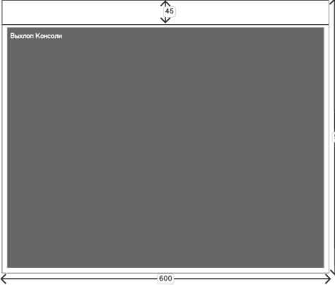
Окно Консоли
